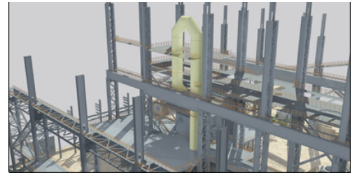
图10 OG系统吊装工艺模拟
