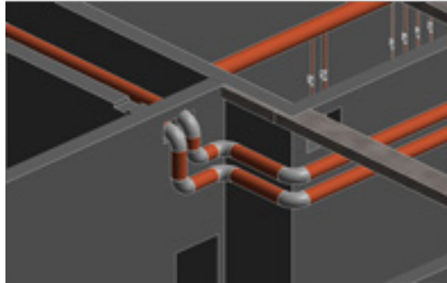
图7上 连铸配水间管道模型 图7下 连铸配水间管道与预留孔洞尺寸存在偏差
