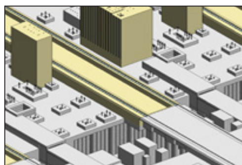
图3上 RH炉基桩和转炉基础存在冲突 图3下 主控楼基础电缆隧道和转炉电缆隧道标高不一致
