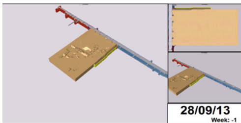
图14 1#2#板坯连铸机施工进度模拟
