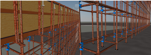
图6 高支模架体参数模型
