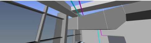
通过更改通风管道标高来解决采暖管道和通风管道碰撞问题 图18 碰撞检查
