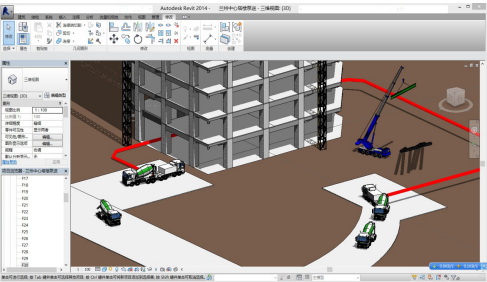
图11 施工现场泵送布置
