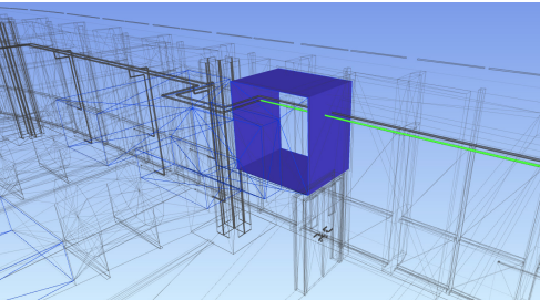
采暖管道与通风管道冲突
