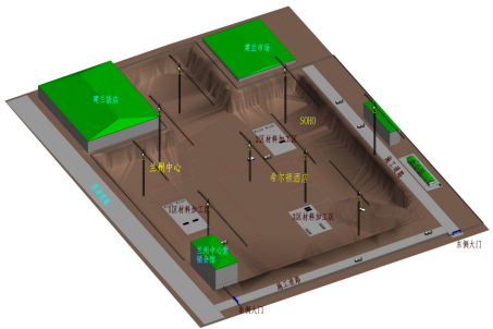
图3 现场三维平面施工布置
