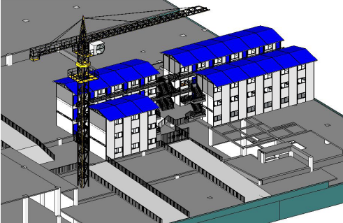
图4 生活区与施工现场合理布置
