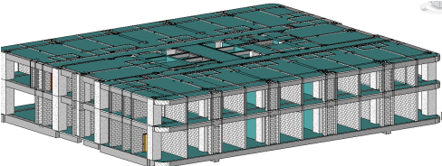
图12 BIM砌筑样板层
