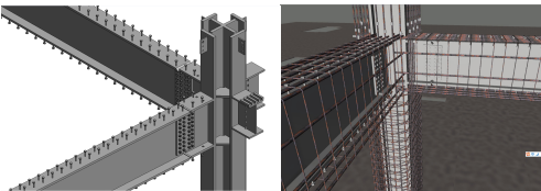
图5 型钢与钢筋混凝土模型
