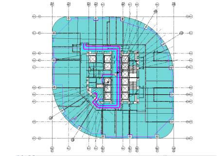
图19 优化设计-原设计管道线路无法满足净空要求
