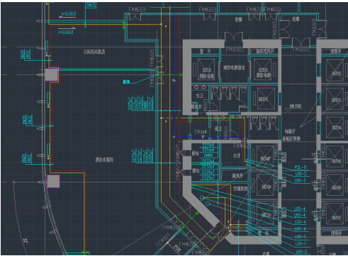
图20 优化设计-调整后的管线布置（满足要求）
