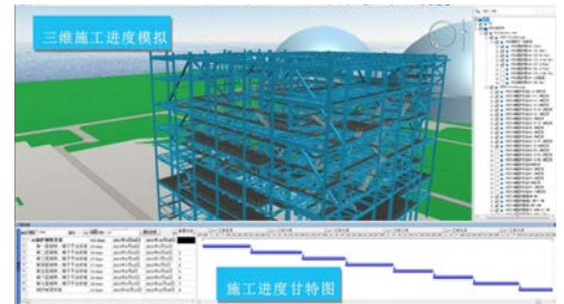
图9 万州工程施工三维可视化应用
