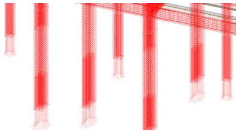
图6 万州工程可视化配筋
