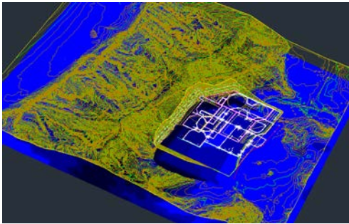
图3 万州工程数字化地形模型
