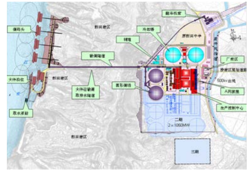
图2 万州工程总平面图
