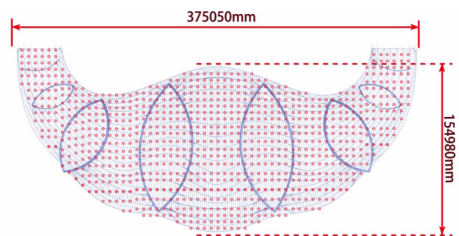
图5 屋盖投影面积大，对接节点多
