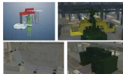
图11 安装工艺模拟
