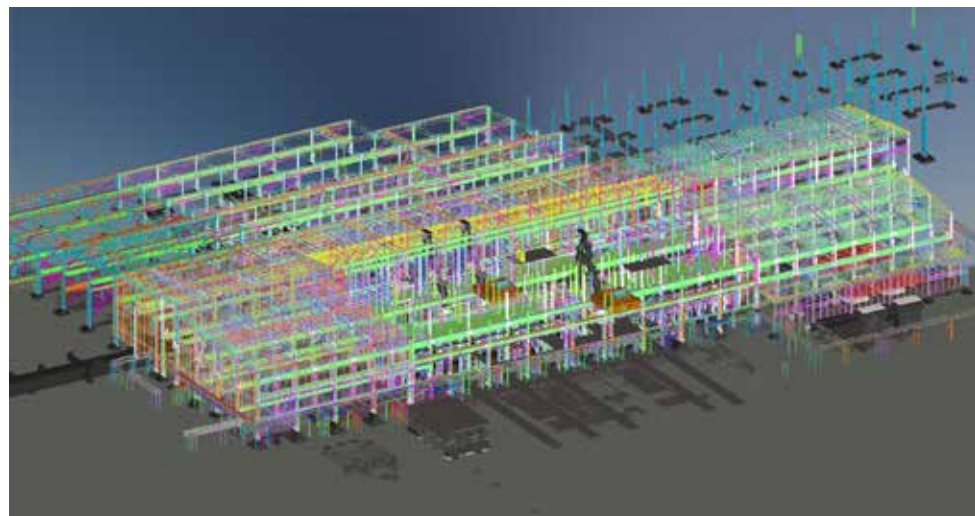
图1 越南河静钢厂总模型
