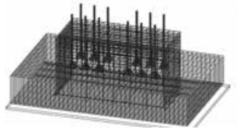
图8下 钢厂柱基础钢筋模型
