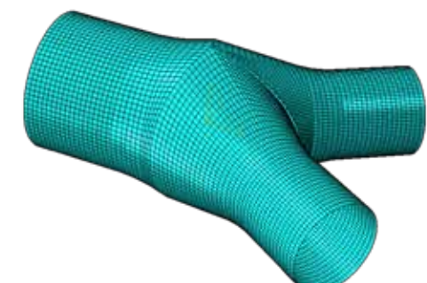
图7 钢岔管有限元网格模型
