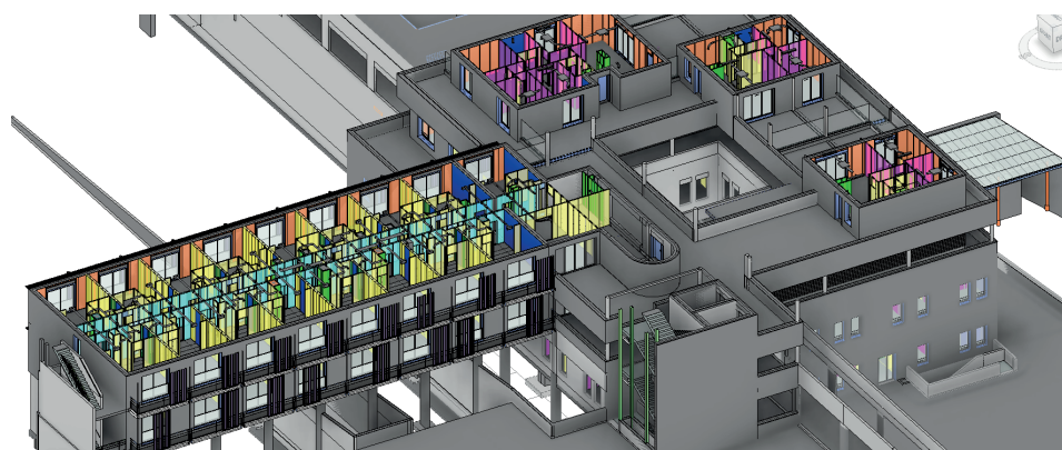
Synthèse de la maquette cloisons avec la maquette fluide pour génération automatique des chevêtres
