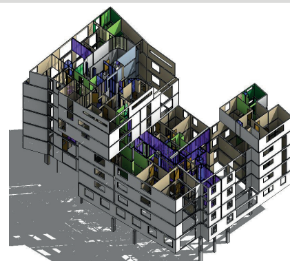
La maquette cloisons d'un projet de logement à Clermont-Ferrand
