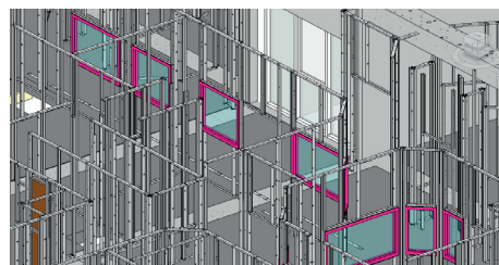
Génération automatique des ossatures suivant les règles programmées pour chaque type de mur
