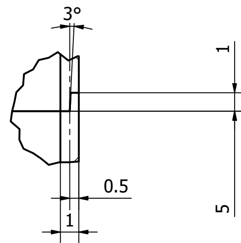
B ( 5 : 1 )
