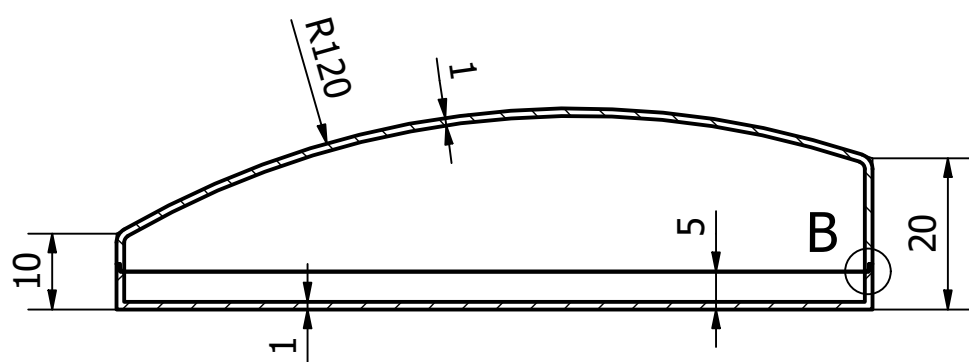
A-A ( 1 : 1 )
